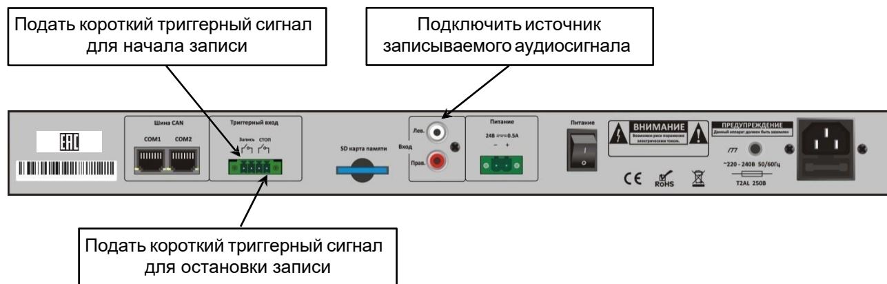
Рис. 4.1. Порядок управления блоком записи сообщений LPA-EVA-RC
